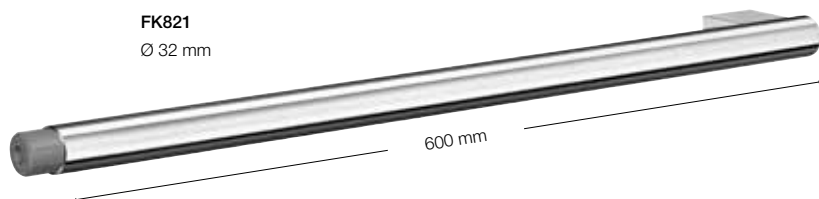
FK820 Haltegriff - Verlängerung 40 cm Fixing point
